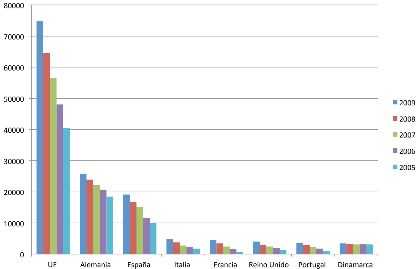
Installierte Windenergie (MW)
